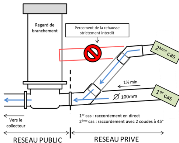
Schéma explicatif du raccordement de vos eaux usées sur le tabouret de branchement
